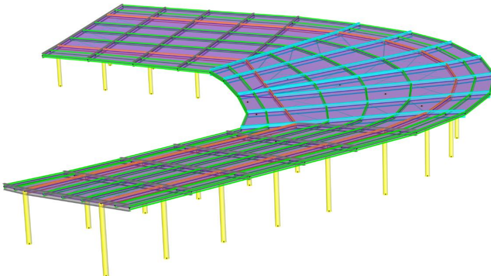
Figura 10 Foto 3 Dimensionale nga programi (struktura)
