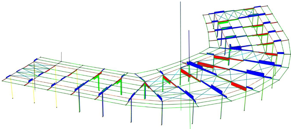
Figura 17 Epyura e forcës prerëse, V
