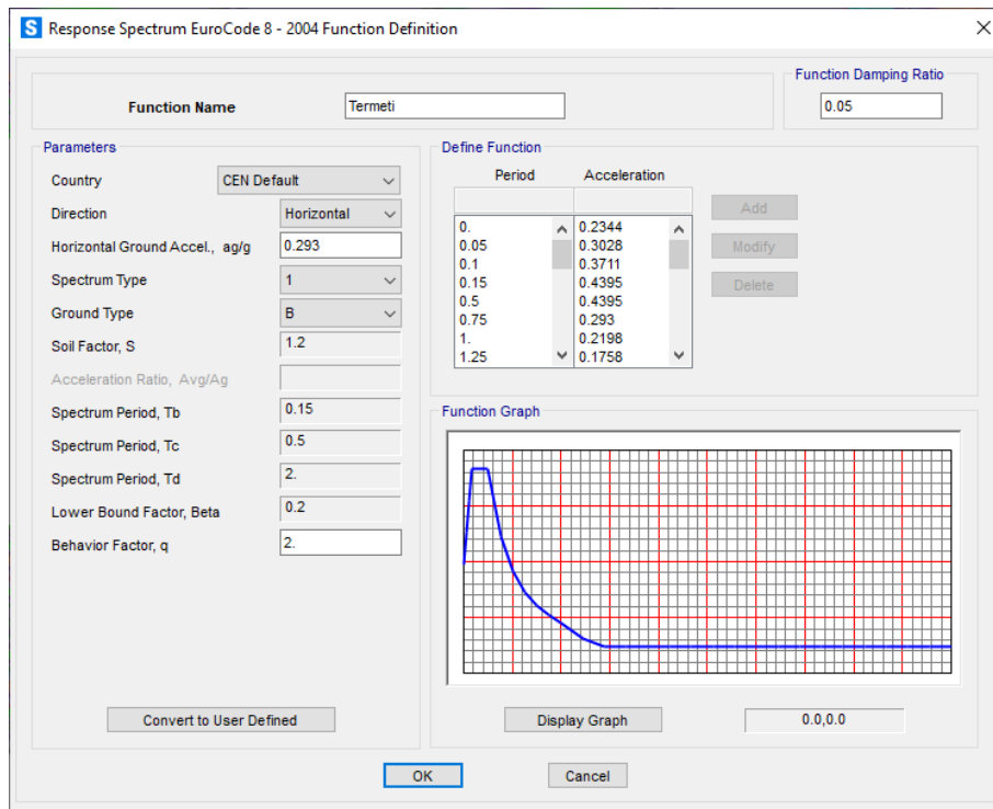
Figura 14 Spektri elastik dhe i projektimit
