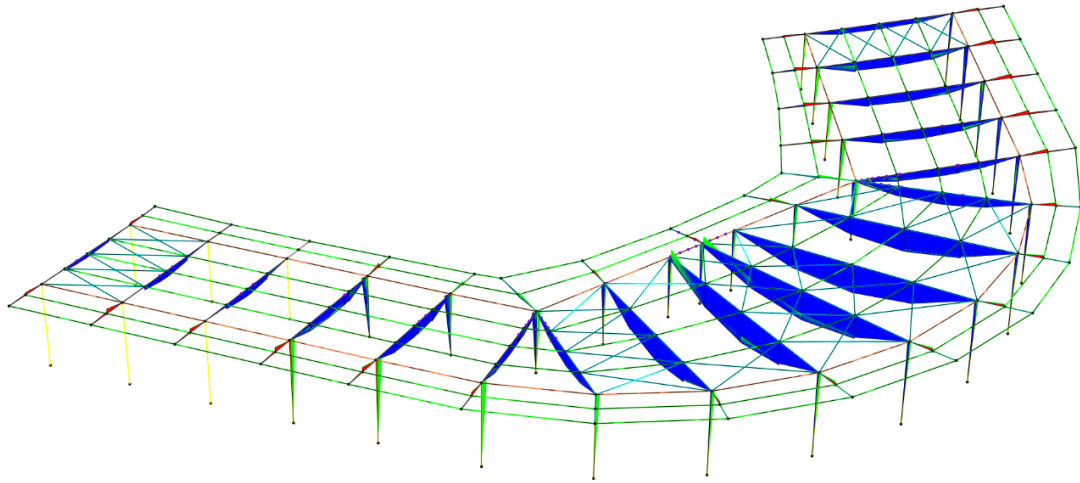
Figura 16 Epyura e momentit përkulës, M
