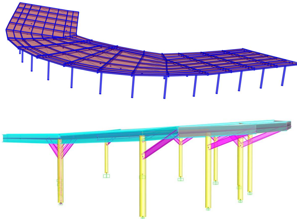
Figura 8 Pamje 3D e strukturës
